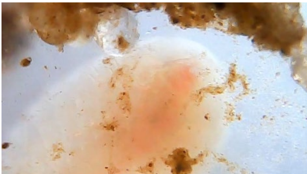
Umgebaute Webcam, Durchlicht
